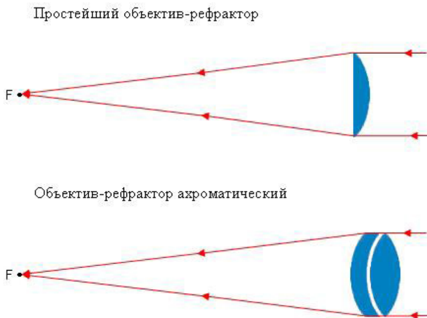
Рис. 2. Рефракторные схемы
