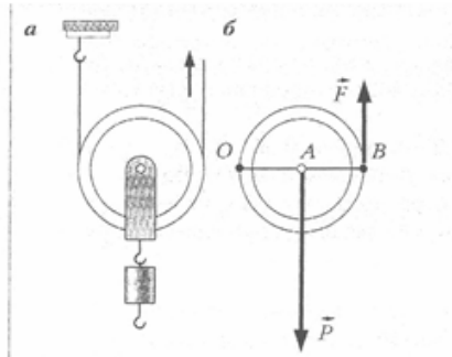
Рис. 144 Подвижный блок, у которого ось вращения перемещается вместе с грузом, можно рассматривать как рычаг второго рода. Такой блок даёт выигрыш в силе в два раза
