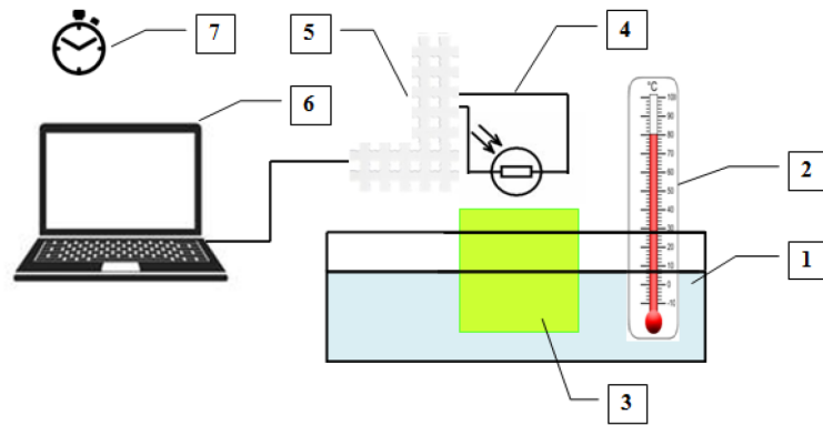
Рис. 1. Экспериментальная установка для исследования реакции с хемилюминесценцией (1 — емкость с водой для поддержания температуры, 2 — термометр, 3 — активированный ХИС, 4 — фоторезистор люксометра, 5 — консольный люксметр ISKRA JS, 6 — компьютер, 7 — таймер)
