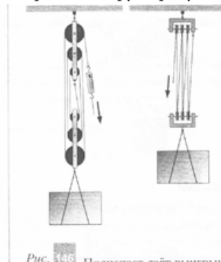
Рис. 146 Полиспаст даёт выигрыш в силе во столько раз, сколько в нём блоков. Изображённые полиспасты имеют по 6 блоков и дают шестикратный выигрыш в силе
