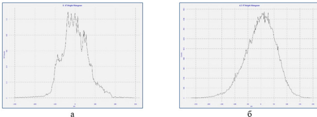
Рис. 4 Гистограммы шероховатости поверхности: а — парафин ( S_a=51,6\text{нм} ), б — воск ( S_a=46,3\text{ нм} )
