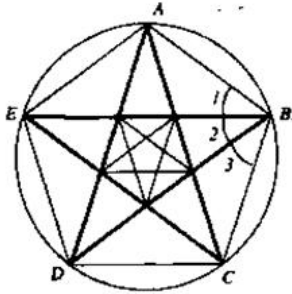
Рис. 5. Свойство 3
