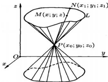
Рис. 2. Коническая поверхность
